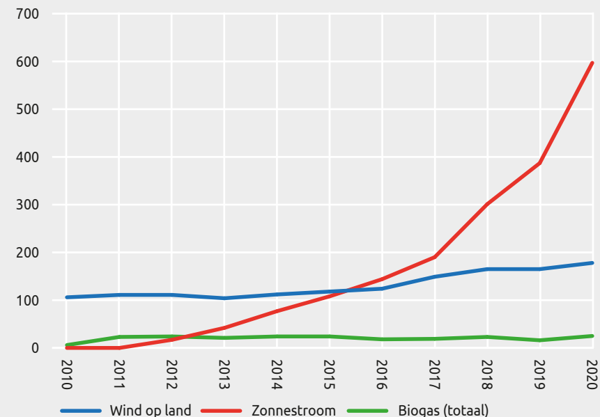
Figuur 26: Ontwikkeling opwek hernieuwbare elektriciteit naar bron in Regio Achterhoek (in TJ), 2010 – 2020
